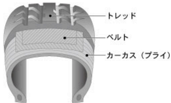
図1●ラジアルタイヤの構造図
