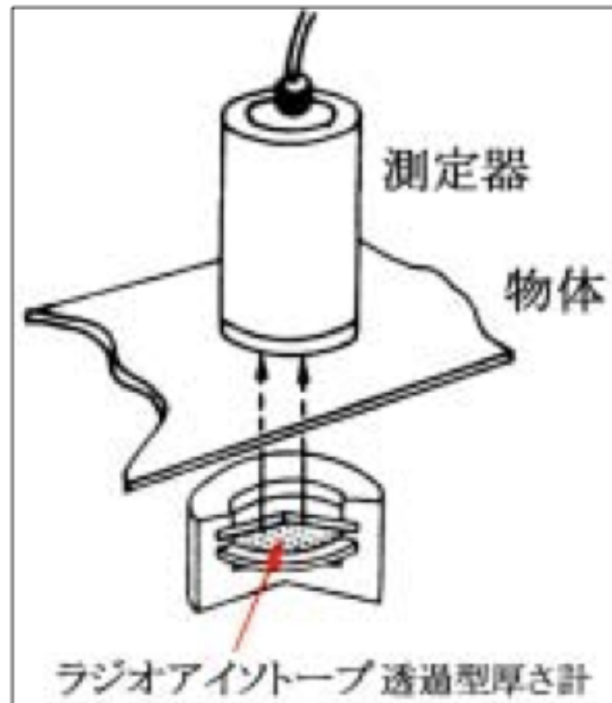
図 8.9.1 厚み計の原理
