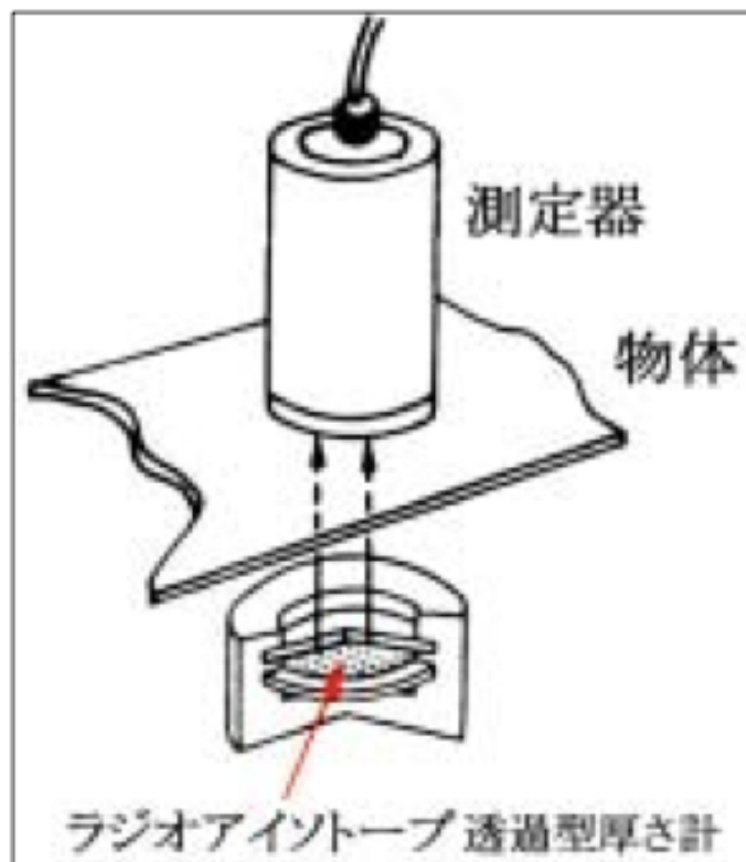
図 8.9.1 厚み計の原理
