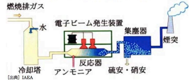
図8.8.1 電子ビームによる石灰燃焼排ガスの処理の原理
