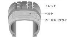
図1=ラジアルタイヤの構造図
