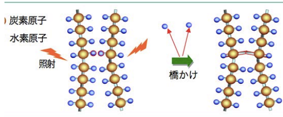
図 8.7.1 放射線によるポリエチレン分子の橋かけの仕組み
